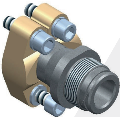
Adaptér HFS s vnějším závitem 2" a SAE připojením
